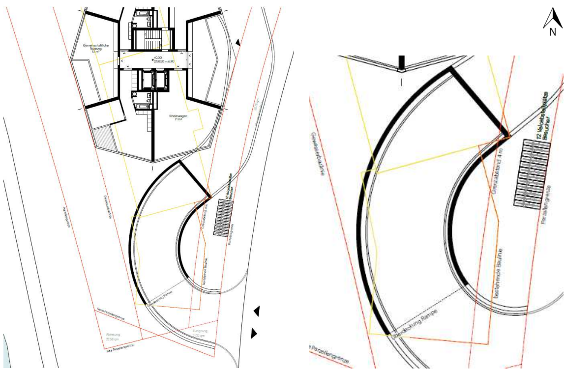
Abbildung 21 Überschreitung Baulinie aufgr. Rampenüberdeckung, rechts vergrößerter Ausschnitt (Quelle: Harry Gugger Studio)
