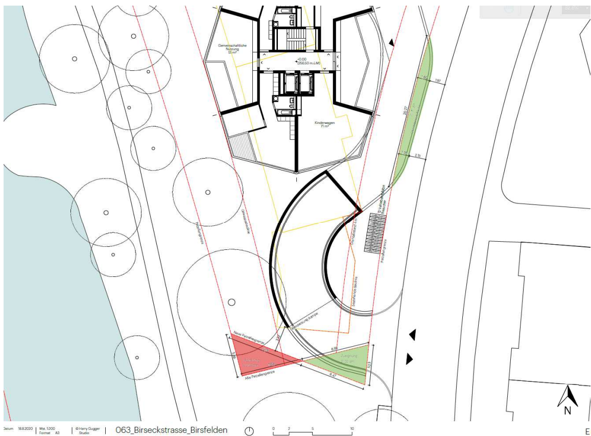
Abbildung 7 Planausschnitt Erdgeschoss Baubereich C und Rampe anschliessendem Durchfahrtsbereich
